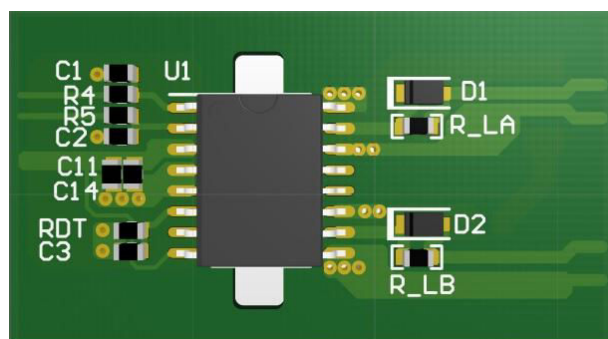
图 11-4. 3D PCB 俯视图
