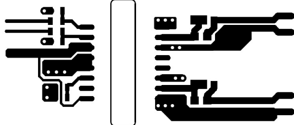
图 11-2. 顶层布线和覆铜
