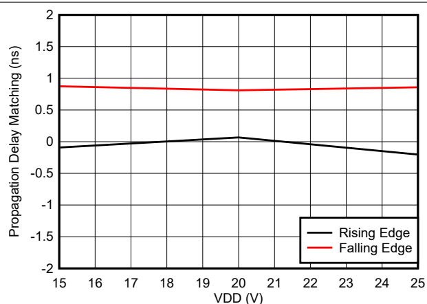
图 6-15. 传播延迟匹配 ( t_{\text{DM}} ) 与 VDD 之间的关系
