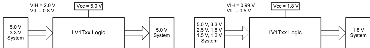
图 8-2. LVxT 升压和降压转换示例
