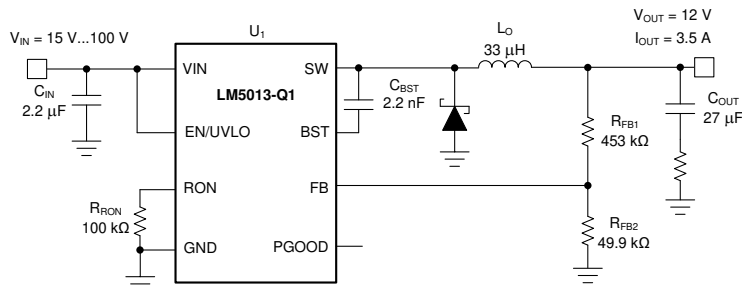
典型应用
