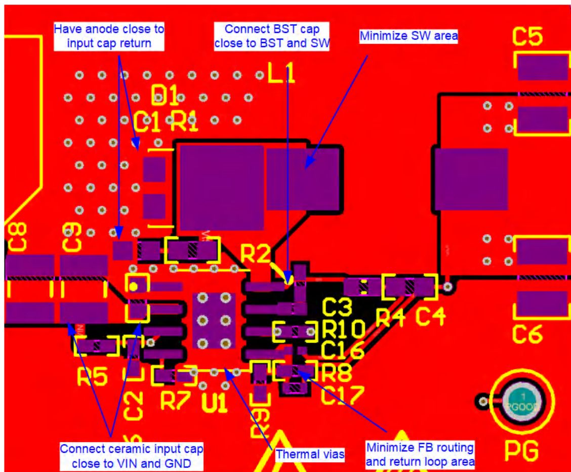
图 10-2. LM5013-Q1 Layout Example
