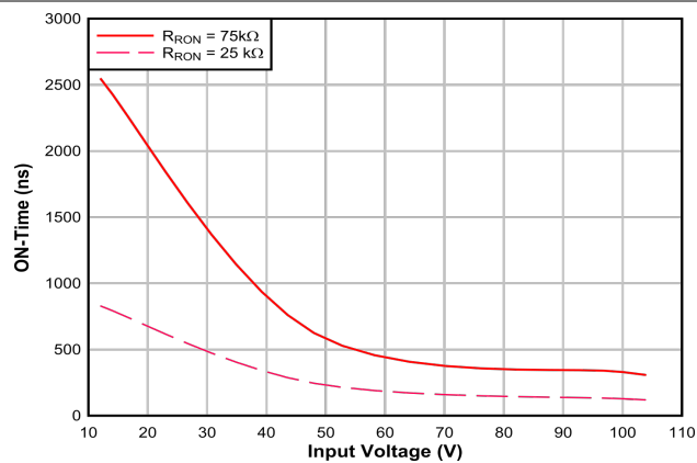
图 6-8. COT On Time Versus V_{IN}
