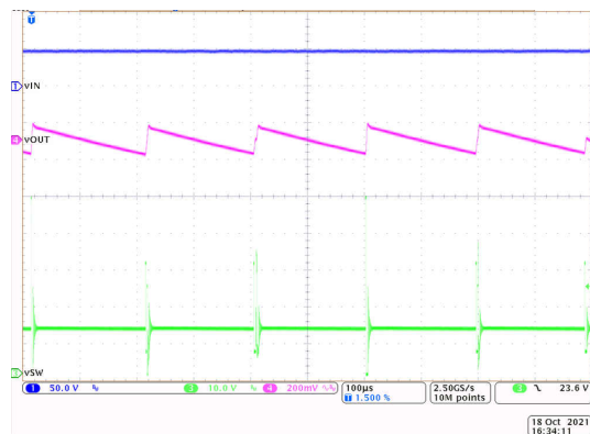
图 8-9. Light-Load Switching
