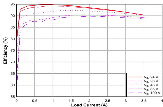
图 6-1. Conversion Efficiency (Linear Scale)
