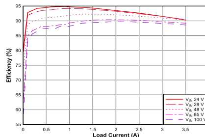
典型应用效率， V_{OUT} = 12V
