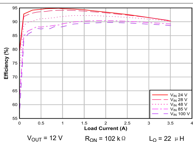
图 8-3. Conversion Efficiency (Linear Scale)
