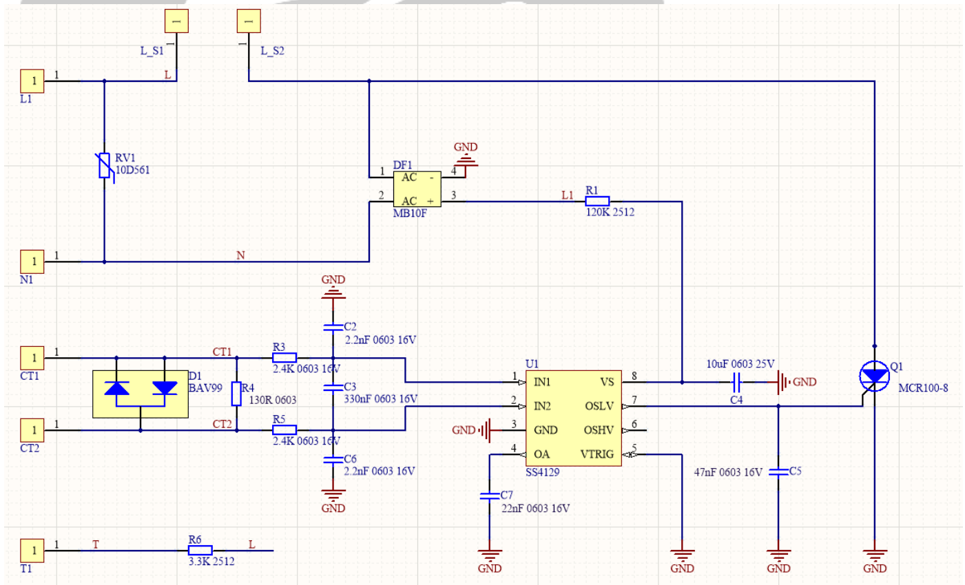
Figure 7. SS4129 典型应用参考电路
