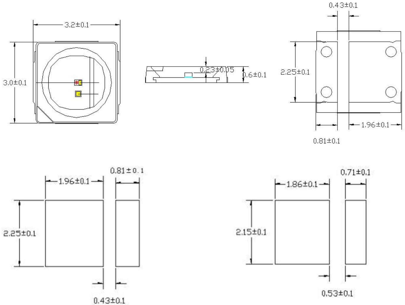
建议焊盘图
