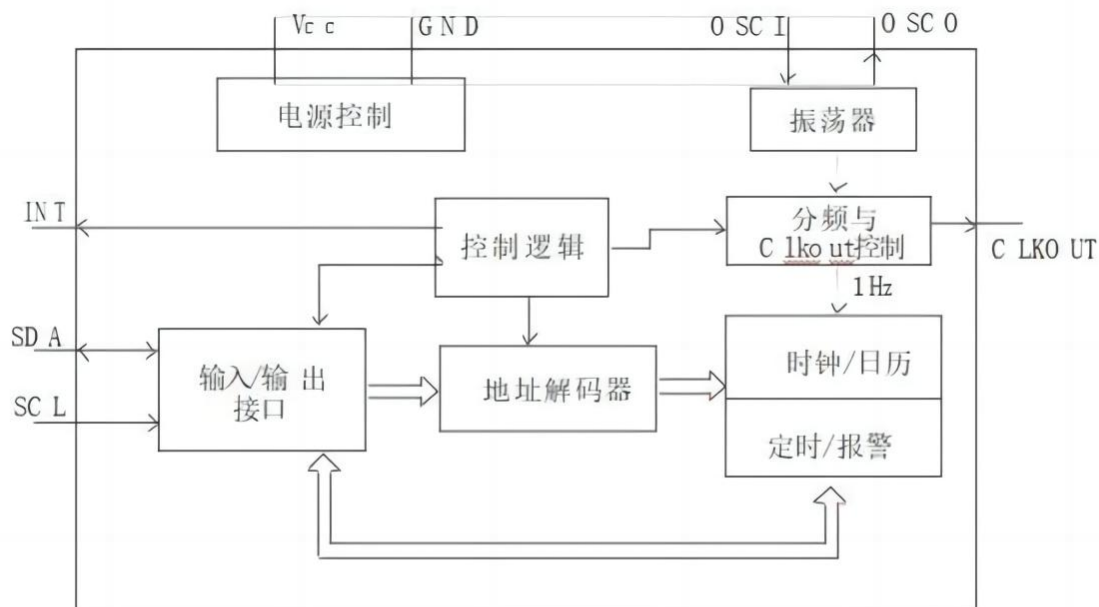
图 2. 方框图
