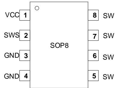
GP7596XA 管脚封装图
