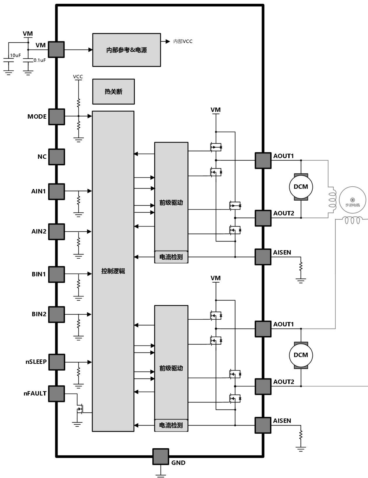
功能模块框图
