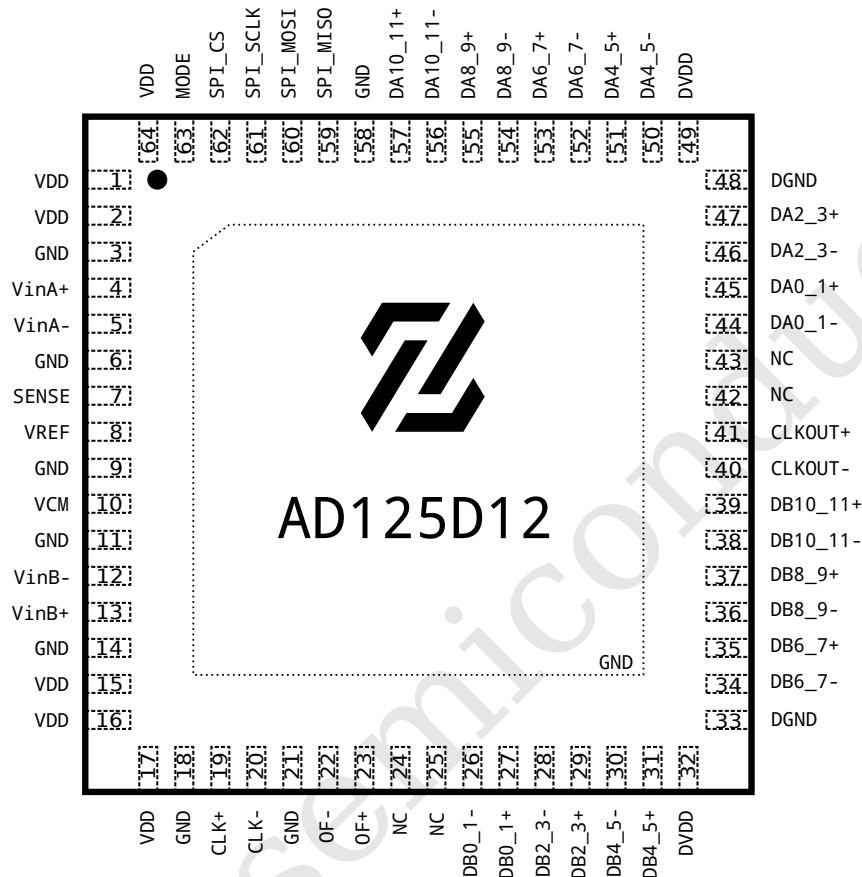
图 4: 正面视图
