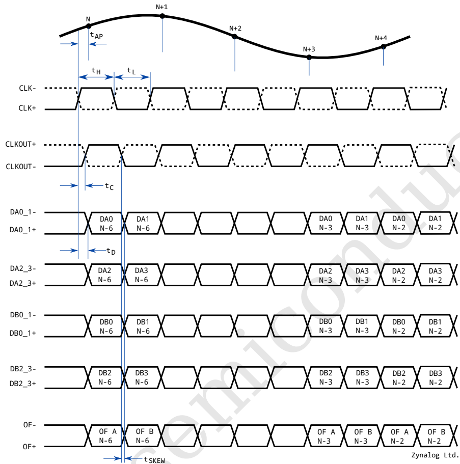
图 5: 数据输出
