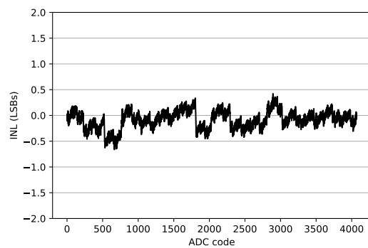
(b) INL
