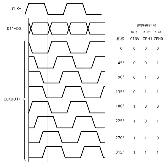
图 13: 相位偏移
