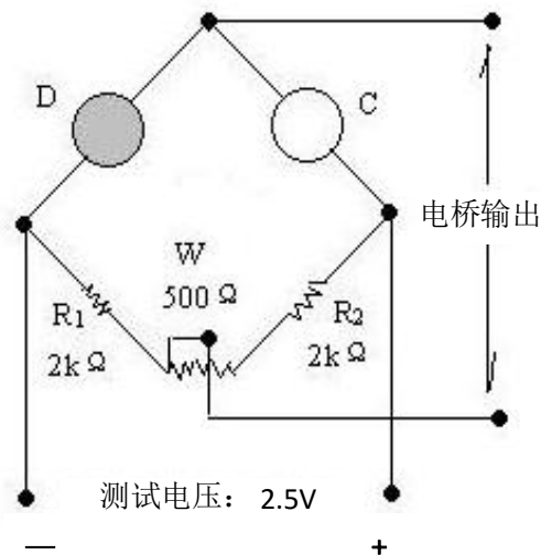
图2：基本测试电路
