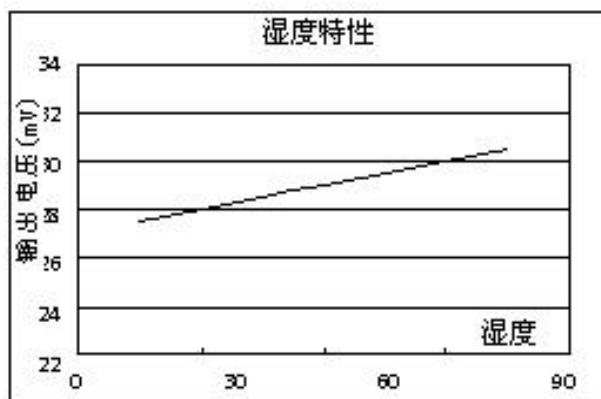
图8：灵敏度湿度特性曲线
