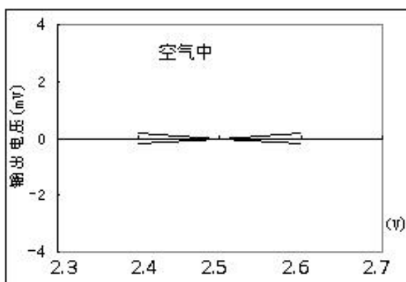
图 9：零点电压波动特性曲线
