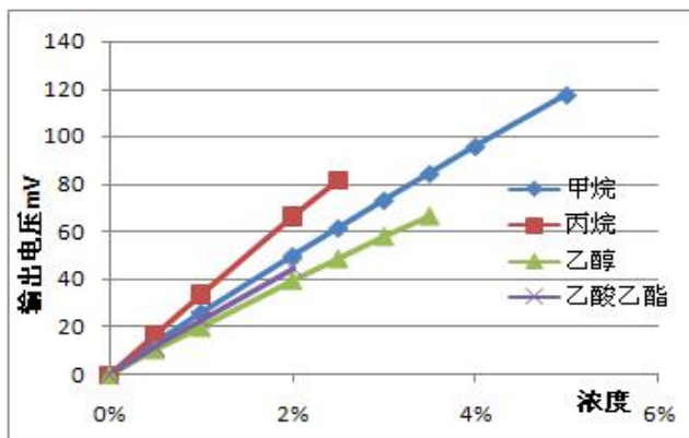
图3：灵敏度曲线
