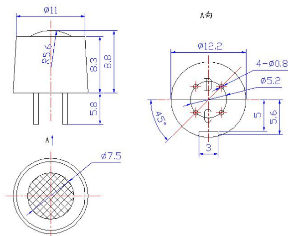
图1：传感器外形结构
