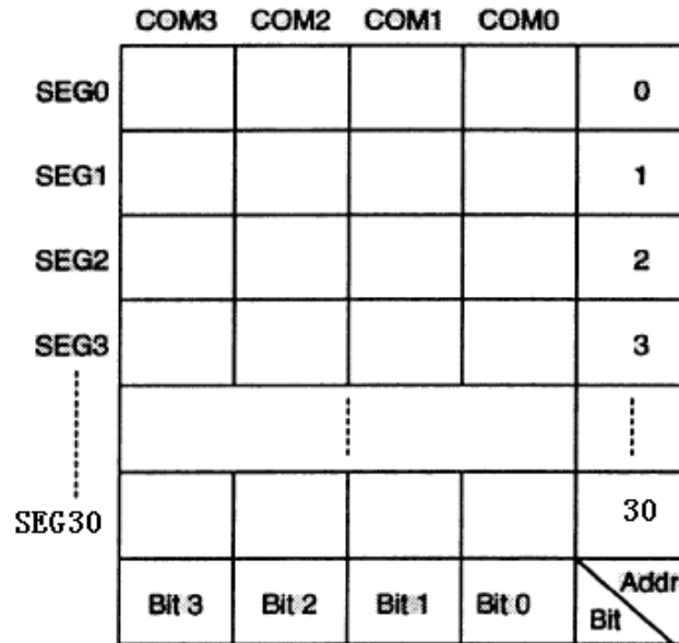
RAM 映象图
